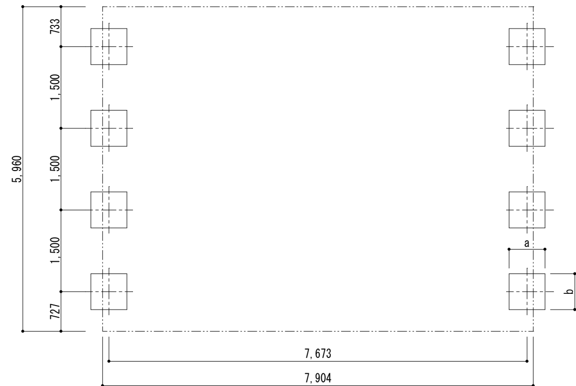
■ 基礎配置図
